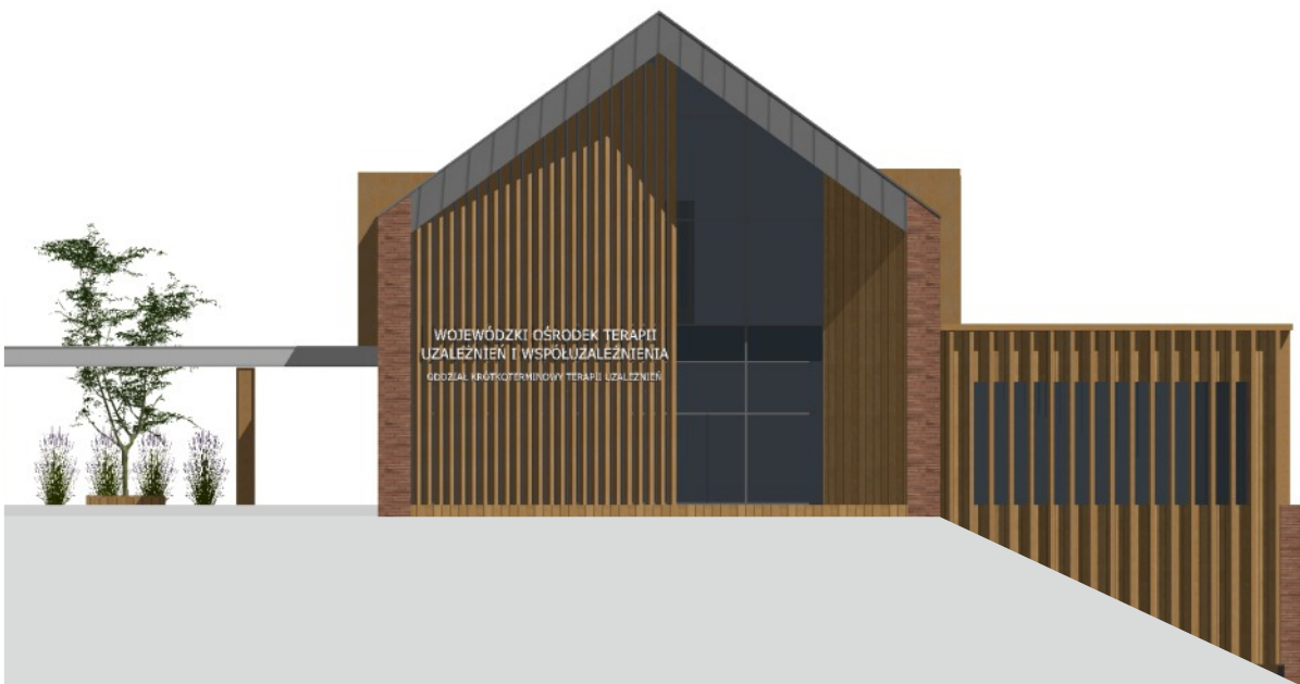
ELEWACJA WSCHODNIA BUDYNKU OKTU
